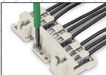
Einbauweise 440V Liegende Schraubmontage auf glatter Oberfläche
