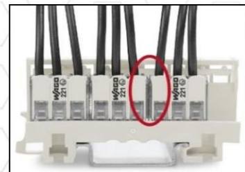
Einbauweise 275V Positionierung der Klemmen im Adapter ohne Distanzelement zwischen den Klemmen
