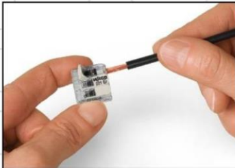
Leiter 11mm abisolieren
