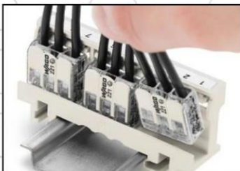
Einrasten der Klemmen in den Befestigungsadapter
